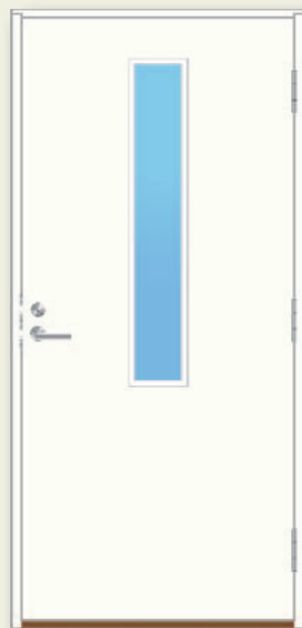
HD 303 Standardstorlekar: 9x20, 9x21, 10x20, 10x21 Standardglas: KLARGLAS. OBS! Dörren har slät insida och dörrbladets tjocklek är 60 mm.
