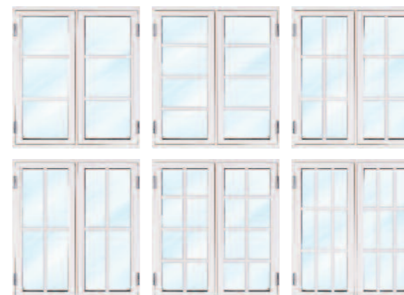
Vårt 2+1 kulturfönster med fastkittad spröjs sett från utsidan
